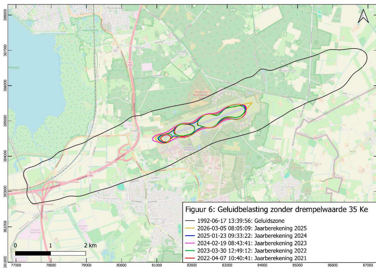
Figuur 6: 35 Ke-geluidbelastingcontouren voor de jaarberekeringen zonder drempelwaarde voor de jaren 2021 tot en met 2025. Zie voor grote afbeelding bijlage D4 op pagina 26
