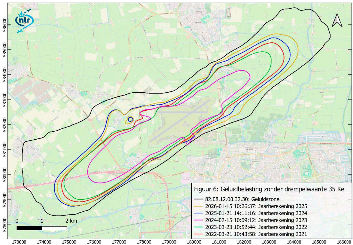
Figuur 6: 35 Ke-geluidbelastingscontouren voor de jaarberekeningen zonder drempelwaarde voor de jaren 2021 tot en met 2025
