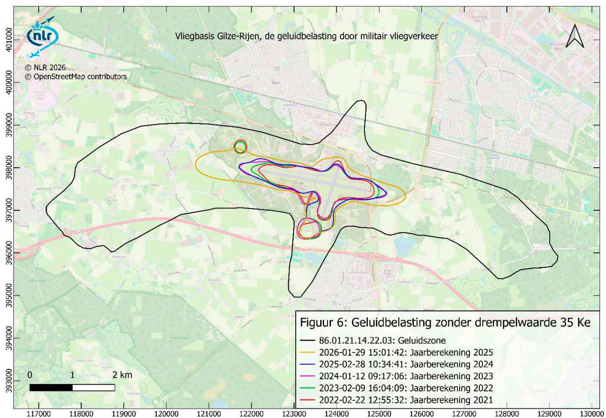
Figuur 6: Ke-geluidbelastingscontouren voor de jaarberekeningen zonder drempelwaarde voor de jaren 2021 tot en met 2025. Zie bijlage D.4 voor grote afbeelding op pagina 27
