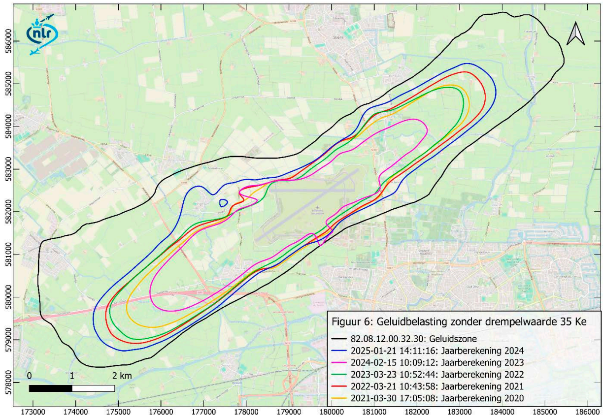
Figuur 6: 35 Ke-geluidbelastingscontouren voor de jaarberekeningen zonder drempelwaarde voor de jaren 2020 tot en met 2024
