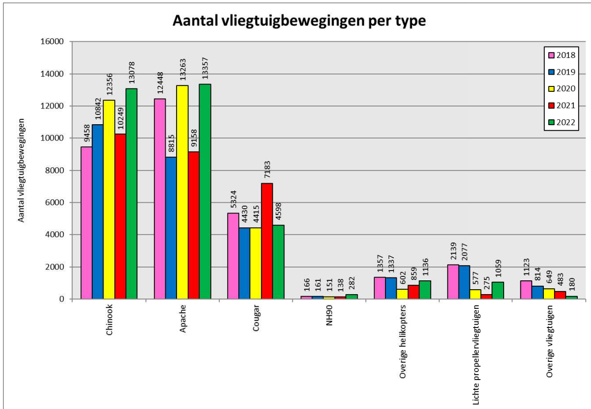
Figuur 5: Werkelijke aantal vliegtuigbewegingen per representatief vliegtuigtype (excl. nachtstraffactor), Vliegbasis Gilze-Rijen
