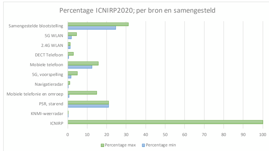
Figuur 4.10 Samengestelde blootstelling de SMART-L in starende modus en met de eigen RF-systemen op 450 m. De balken geven de minimale (blauw) en maximale (groen) te verwachten elektrische veldsterkte weer. Beide waarden worden vergeleken met de ICNIRP2020-richtlijn. Lager dan 100% betekent dat aan de richtlijn voldaan wordt.
